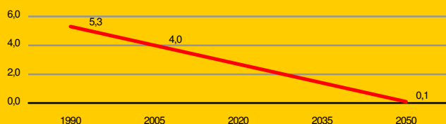
Figur 3. Klimatmålen 2005-2050 jämfört med basåret 1990 16
