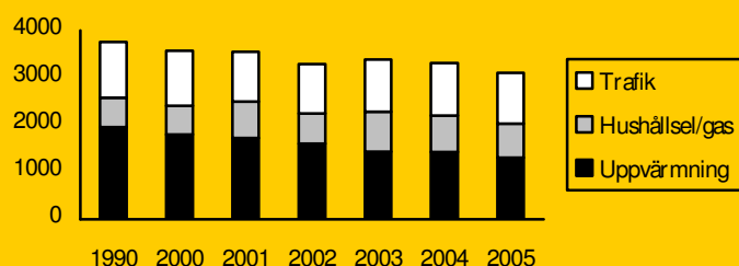
Figur 4. Sammanlagda utsläpp av växthusgaser, tusen ton CO 2 -ekvivalenter, i Stockholms stad mellan 1990 och år 2005. Normalårskorrigerade. År 1990 och 2005 var ovanligt varma år 17
